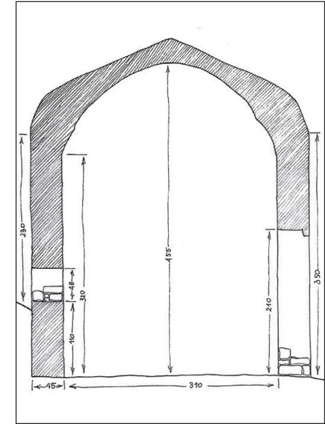
Schemazeichnung des Reinheimer Trullo
