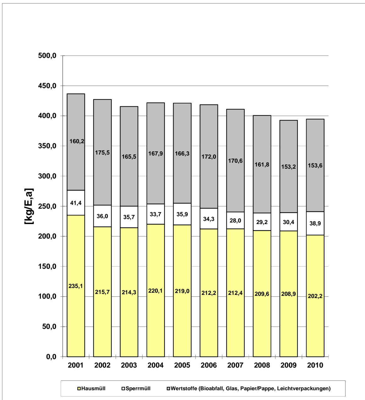
Abb. 4: Spezifisches Brutto-Abfallaufkommen
